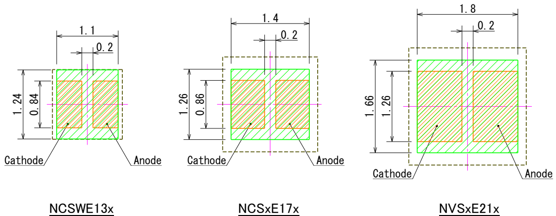
図 9. NSMD 方式の推奨ランドパターン
