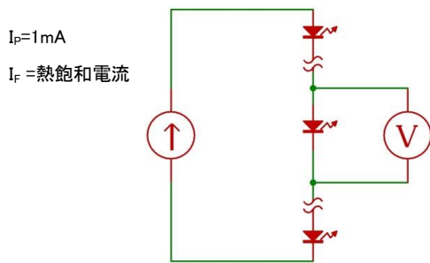
図 16. 測定回路
