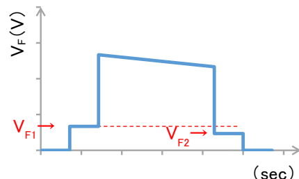
図 18. 測定電圧
